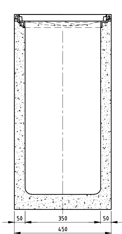
Zijaanzicht
