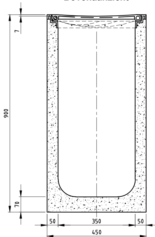
Vooraanzicht
