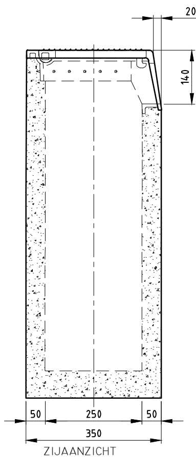
ZIJAAANZICHT
