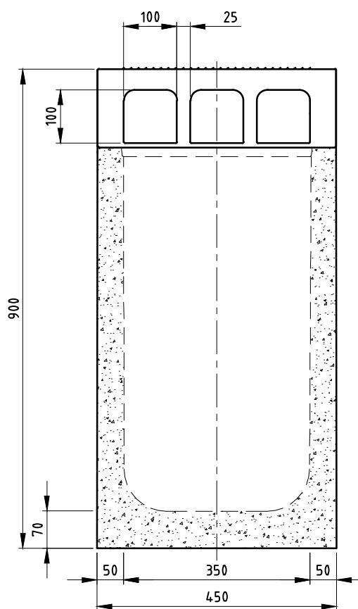
VOORAANZICHT
