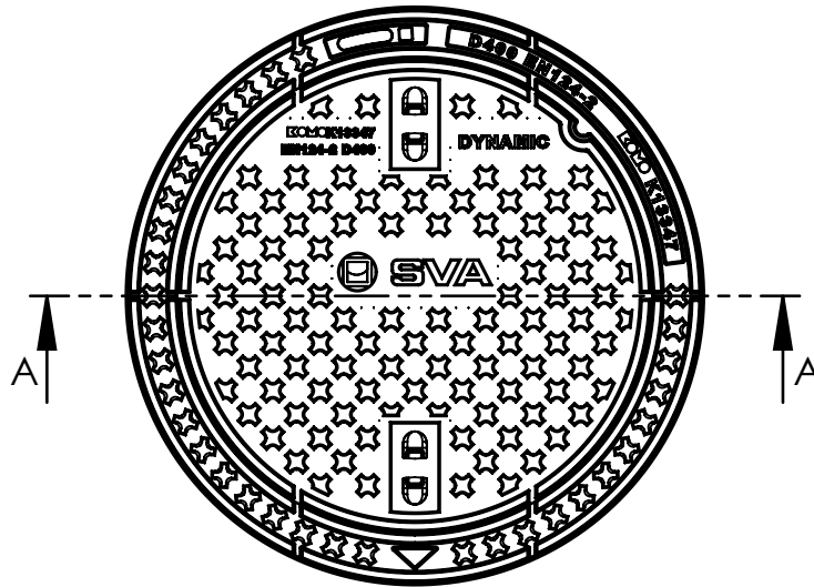
Deksel met ontluchtingsgaten in de haalkommen
