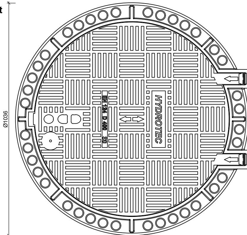
Bovenaanzicht
