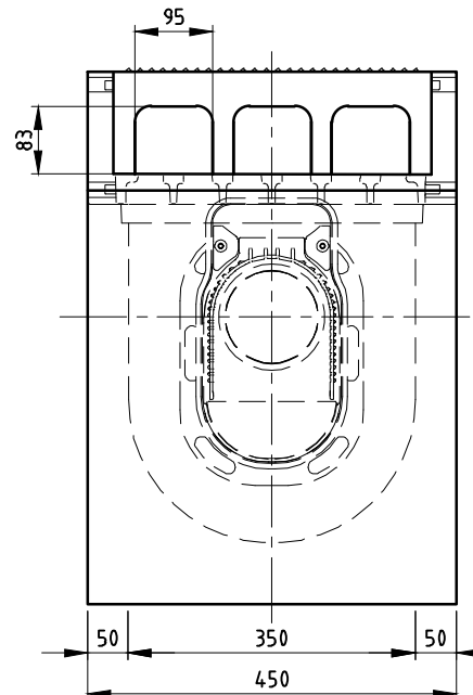
Vooraanzicht
