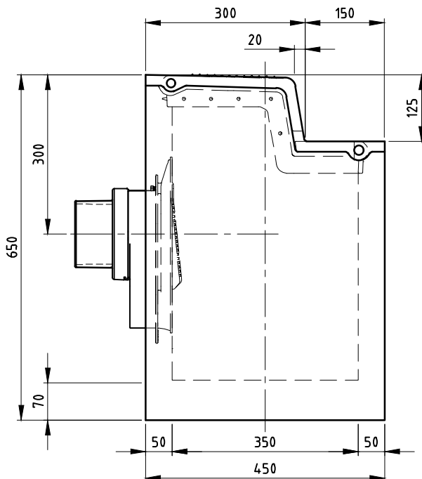
Zijaanzicht
