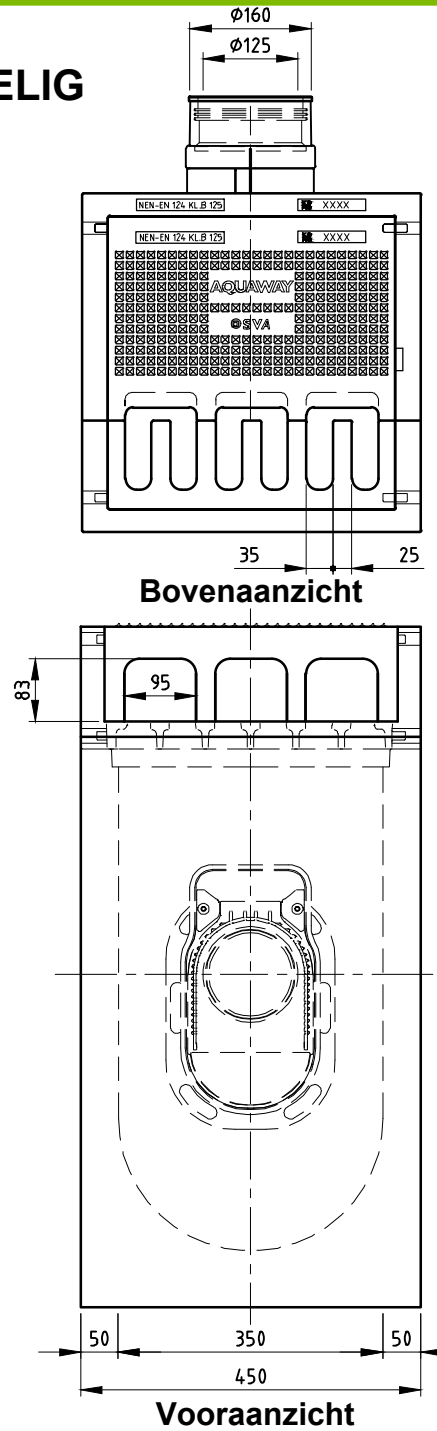
Scharnierende putklep
