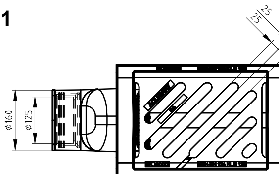
Bovenaanzicht
