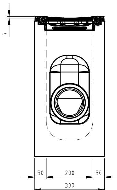
Zijaanzicht
