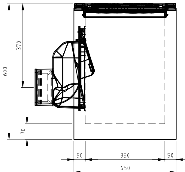
Vooraanzicht
