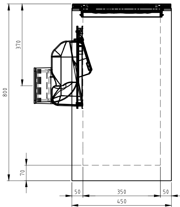
Vooraanzicht
