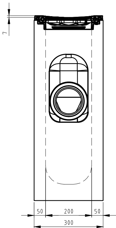
Zijaanzicht
