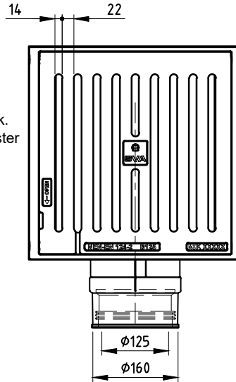
BOVENAANZICHT
