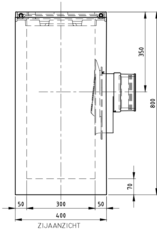
ZIJAANZICHT
