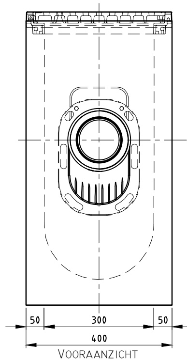
VOORAANZICHT
