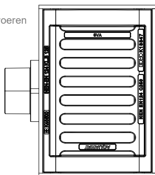
Bovenaanzicht
