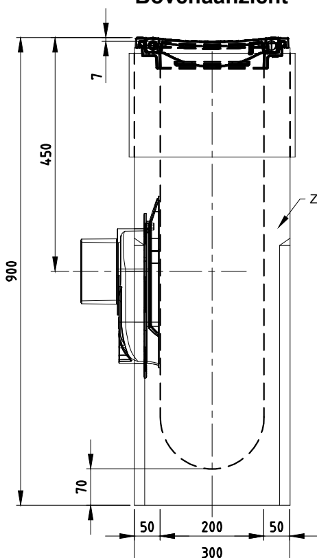
Vooraanzicht
