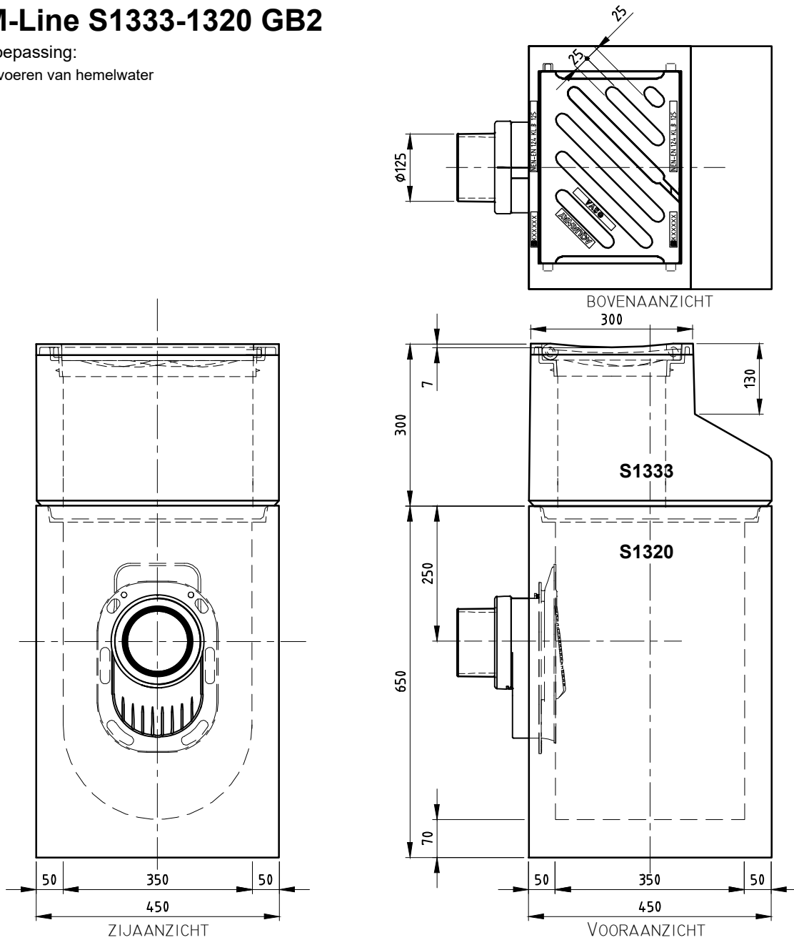
Scharnierende putklep
