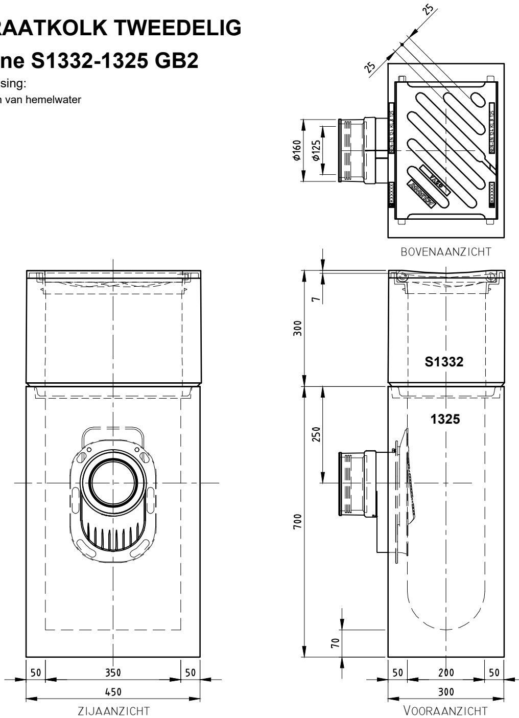
Scharnierende putklep
