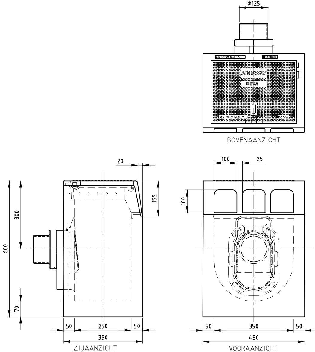
Scharnierende putklep
