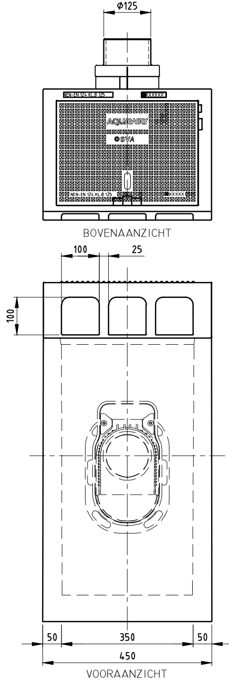
Scharnierende putklep
