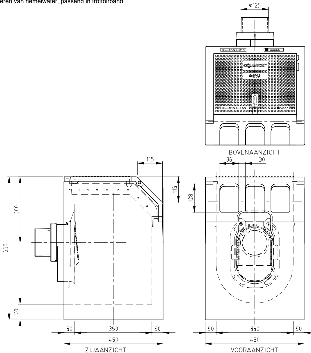
Scharnierende putklep
