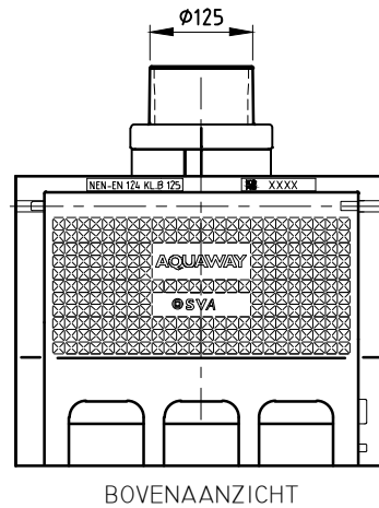
BOVENAANZICHT
