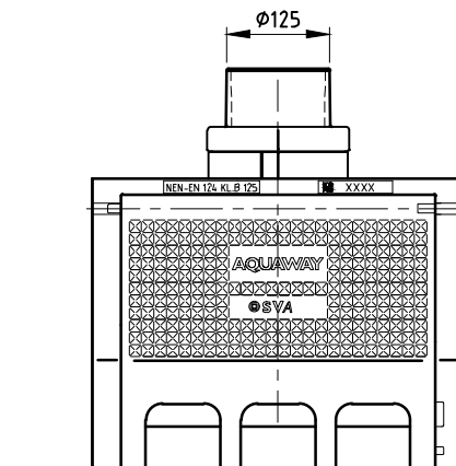
BOVENAANZICHT
