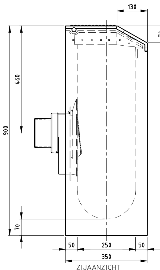
ZIJAANZICHT
