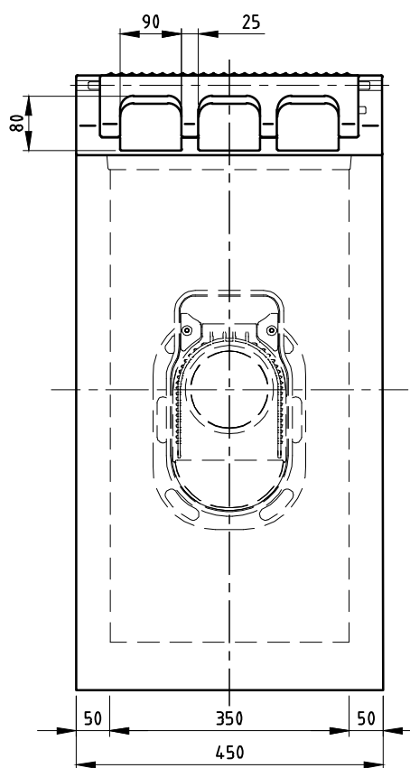
VOORAANZICHT
