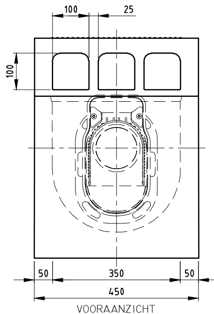
Waaierdeksel C250
