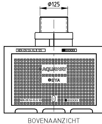
BOVENAANZICHT
