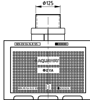
BOVENAANZICHT
