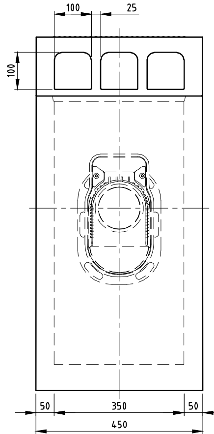
VOORAANZICHT
