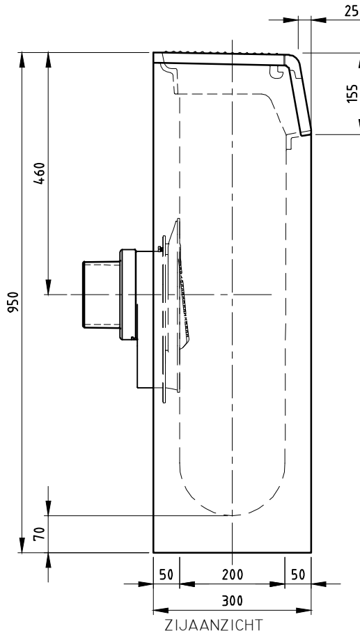
ZIJAANZICHT
