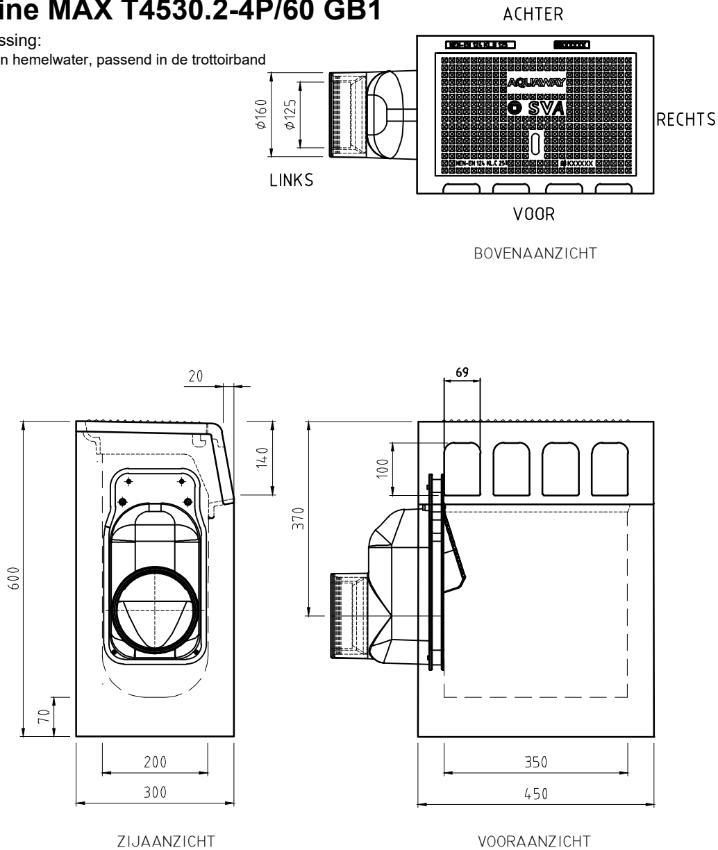
Scharnierende putklep
