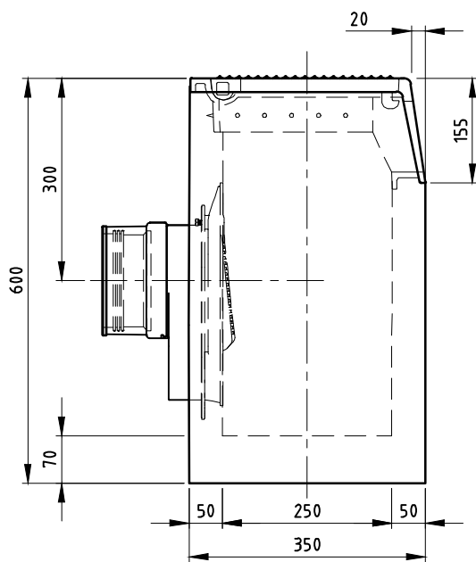
ZIJEAANZICHT
