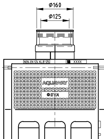
BOVENAANZICHT
