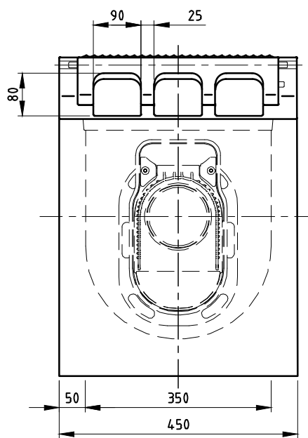
VOORAANZICHT
