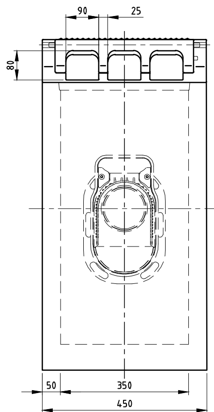
VOORAANZICHT
