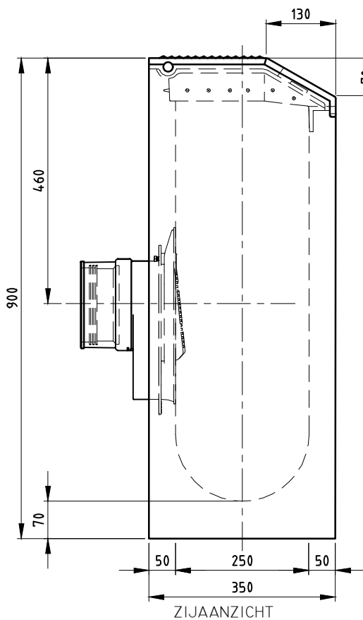
ZIJAANZICHT
