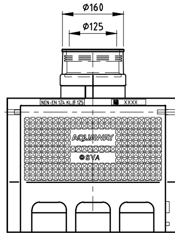
BOVENAANZICHT
