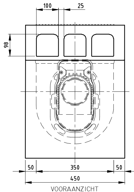
VOORAANZICHT
