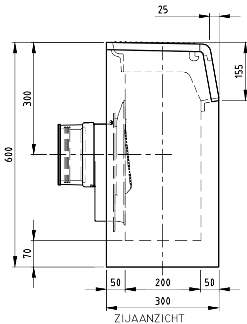
ZIJAANZICHT
