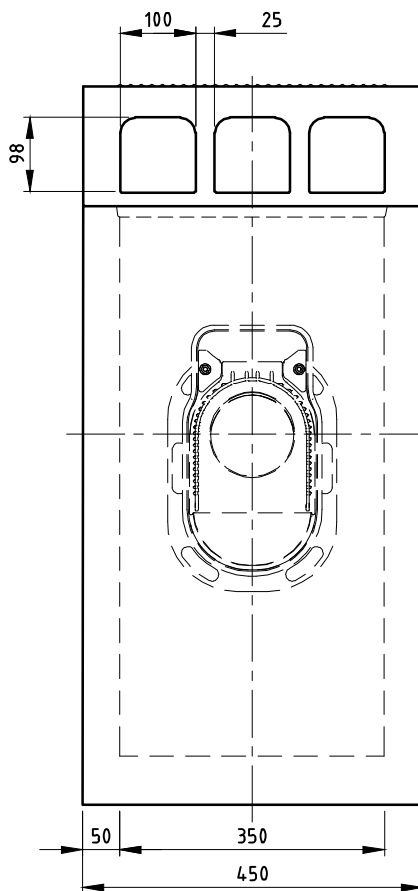
VOORAANZICHT
