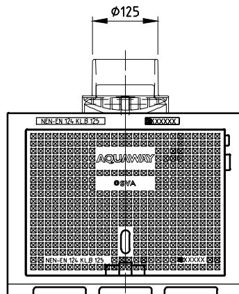
BOVENAANZICHT
