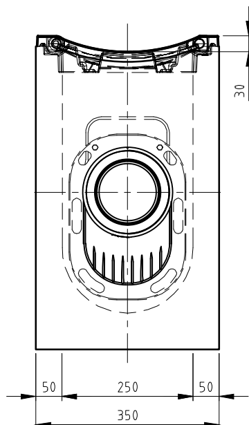
ZIJAANZICHT
