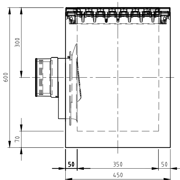
VOORAANZICHT
